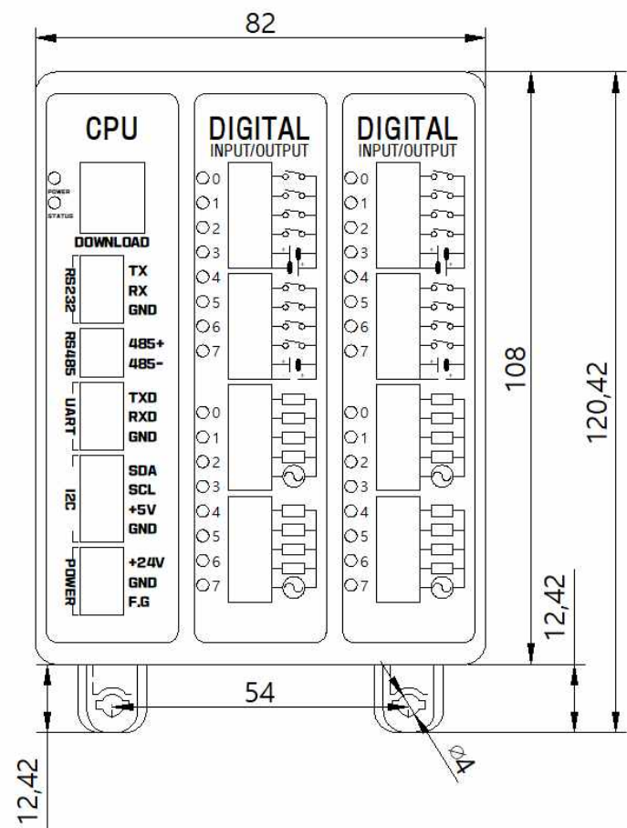
□ DIMENSION ( 클립 열었을 때 / 딘 레일 체결 후 )
