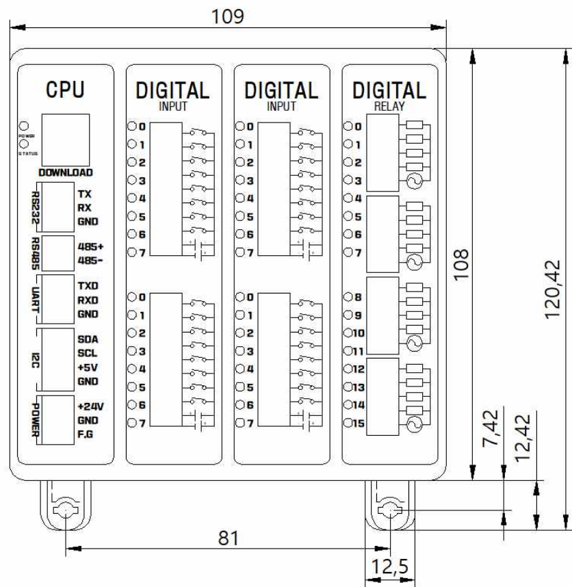
□ DIMENSION ( 클립 열었을 경우 )
