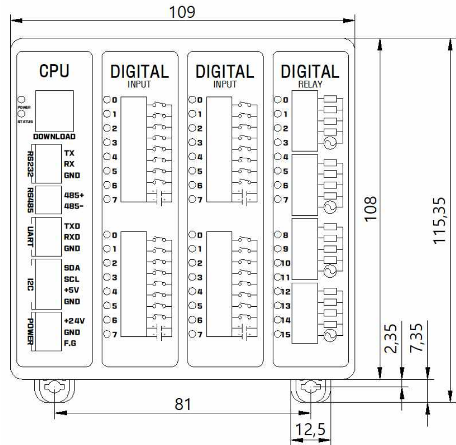
□ DIMENSION ( 클립 닫았을 경우 )
