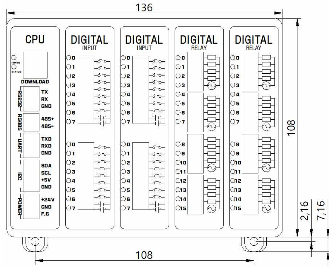
□ DIMENSION ( 클립 닫았을 경우 )
