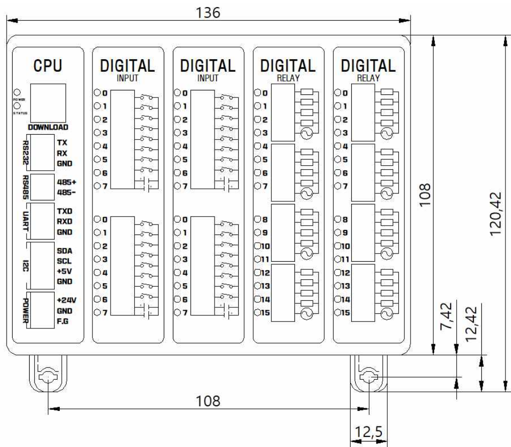
□ DIMENSION ( 클립 열었을 경우 )
