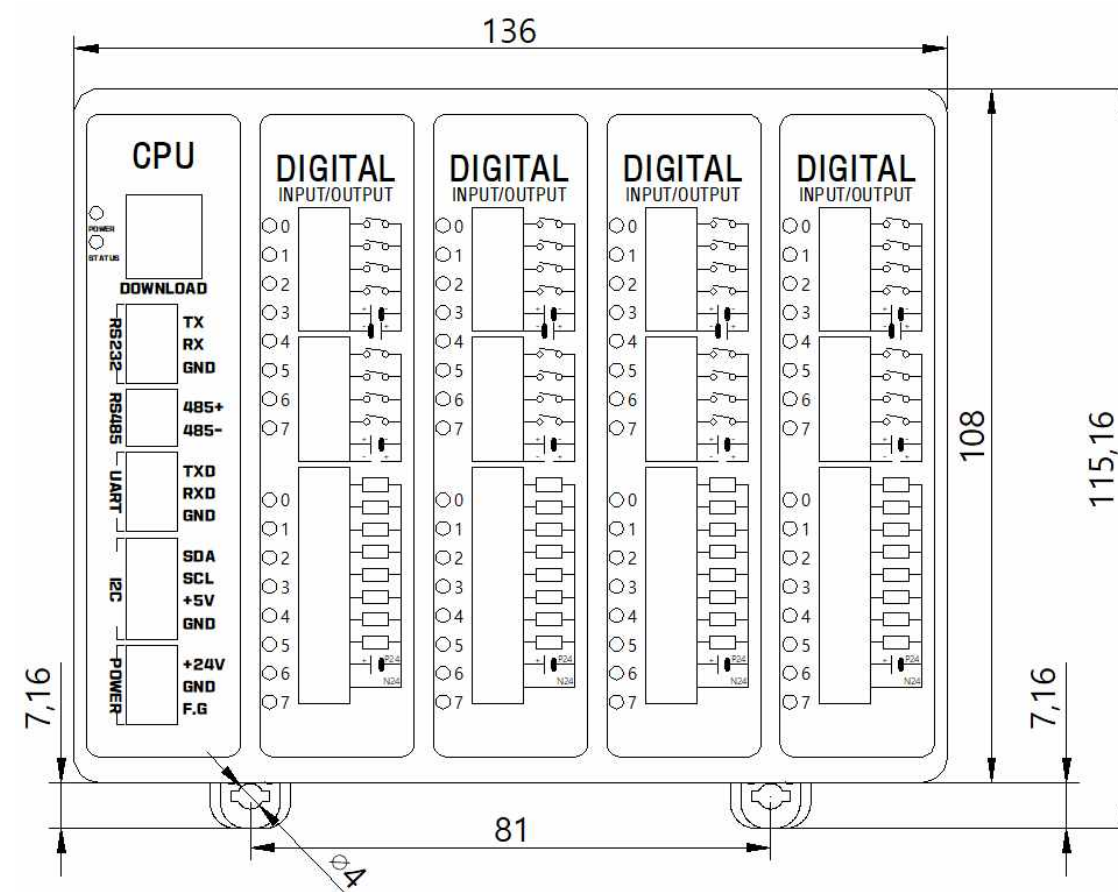
❑ DIMENSION ( 클립 단았을 경우 )
