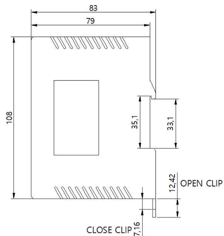
□ DIMENSION ( 클립 열었을 때 / 딥 레일 체결 후 )
