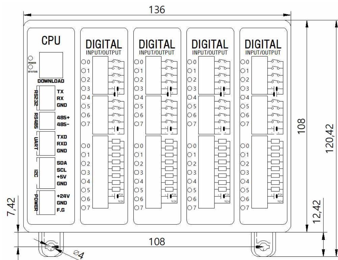
❑ DIMENSION ( 클립 열었을 경우 )
