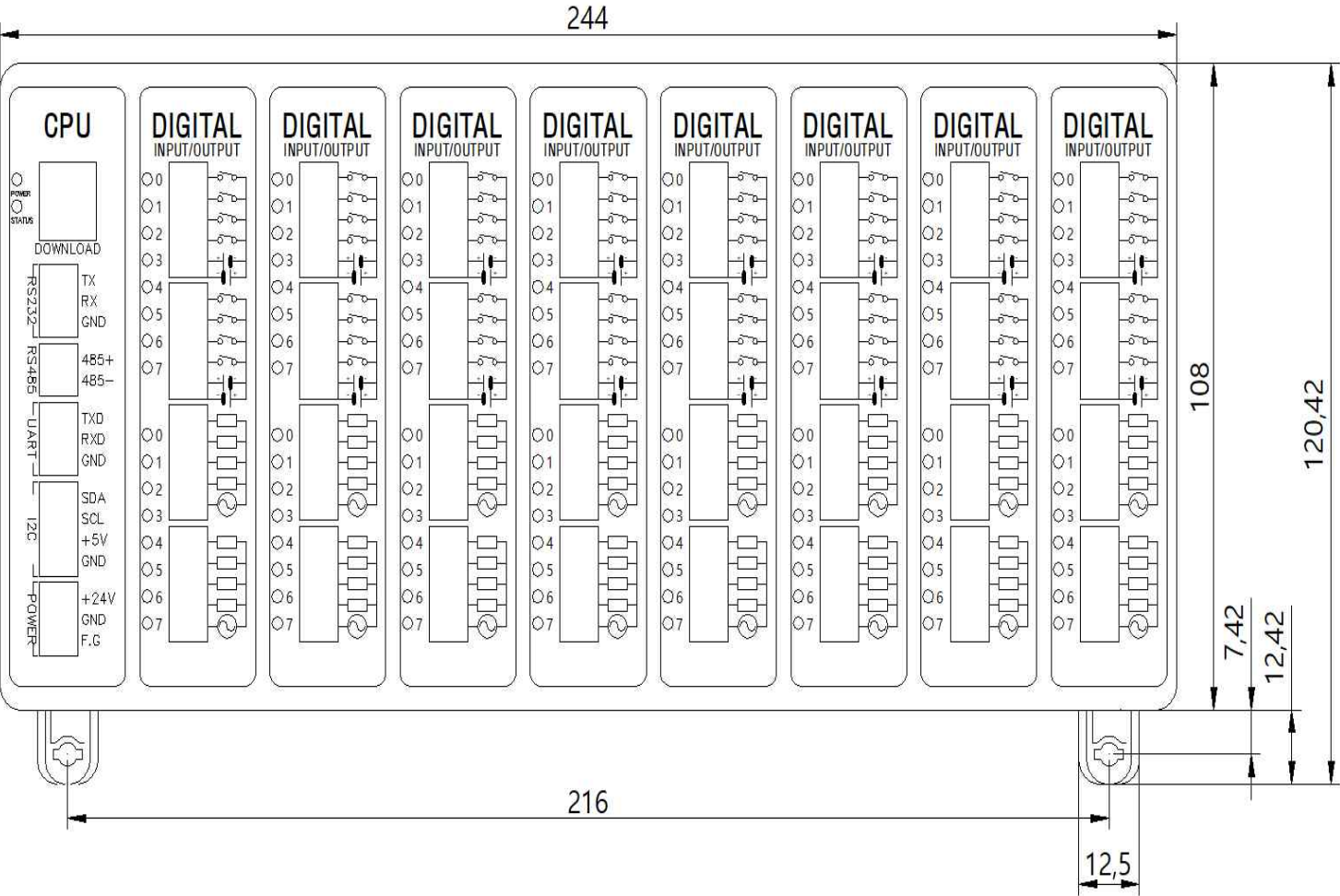
□ DIMENSION ( 클립 열었을 때 / 딘 레일 체결 후 )
