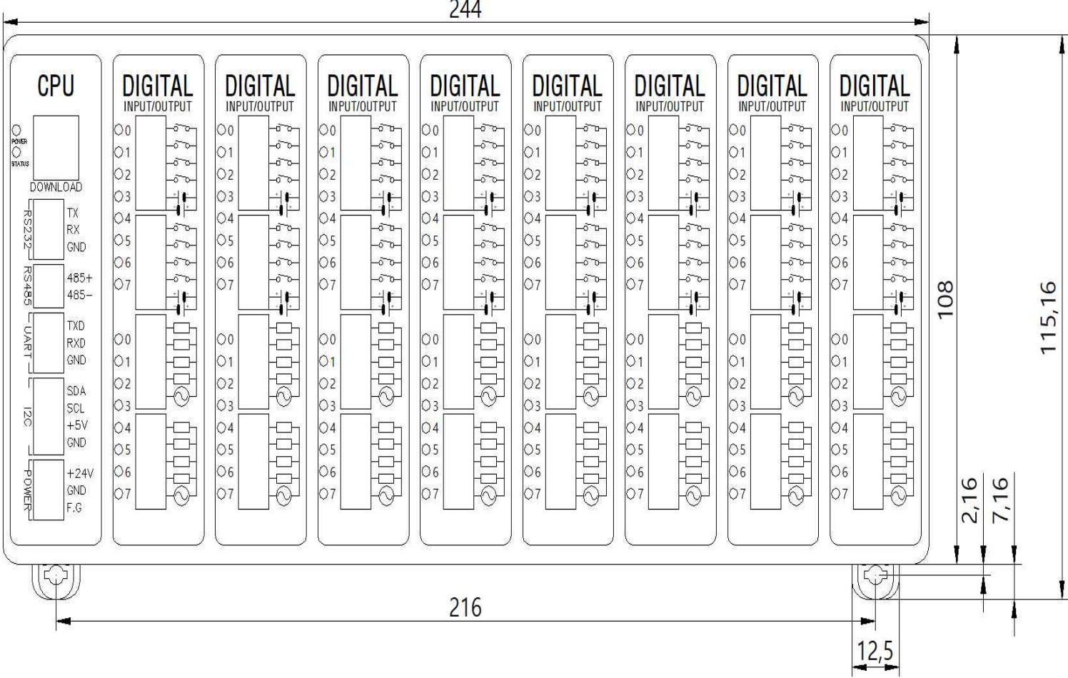
□ DIMENSION ( 클립 닫았을 경우 )
