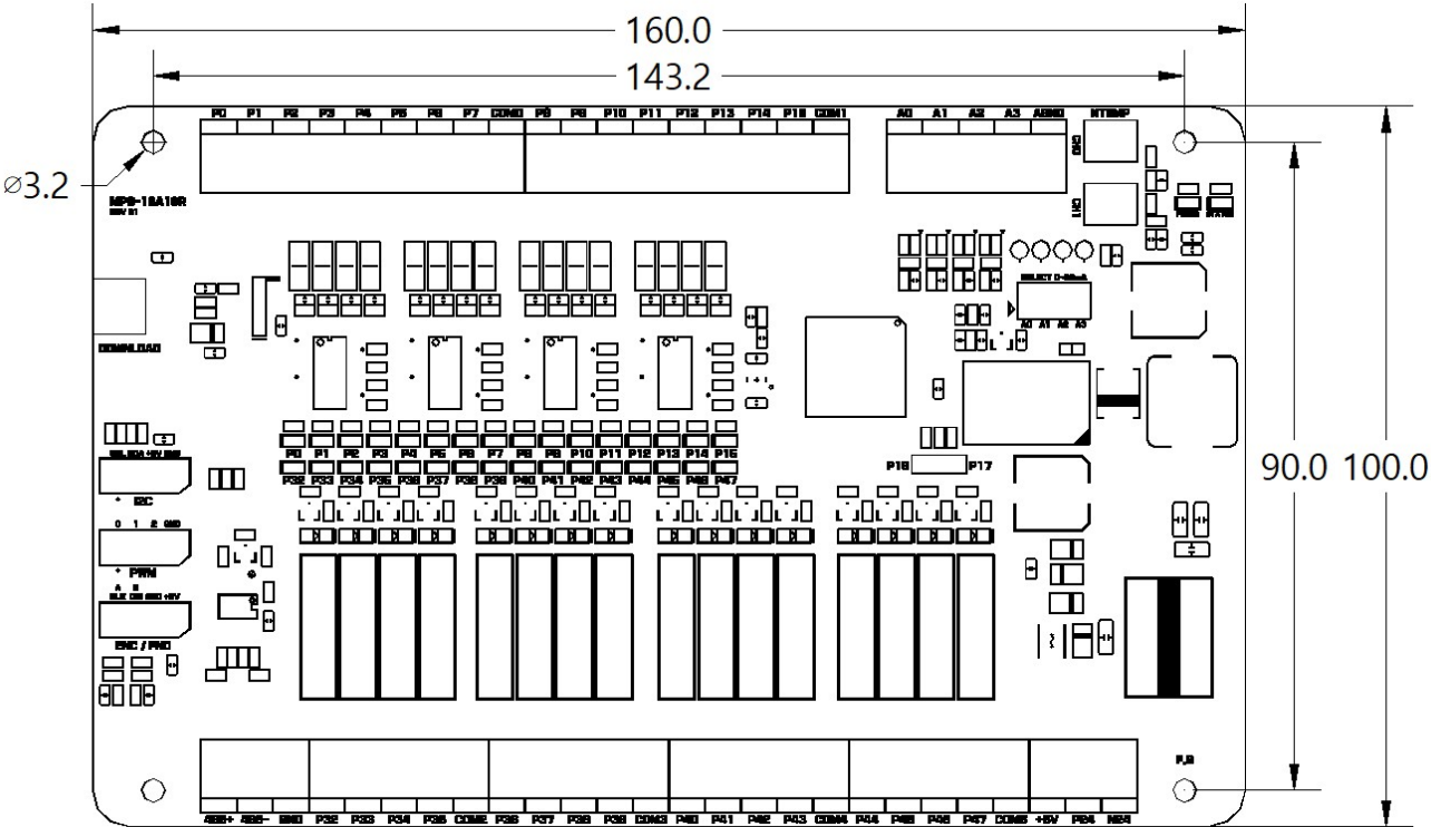
□ DIMENSION ( PCB / 단레일 사용하지 않을 경우 )
