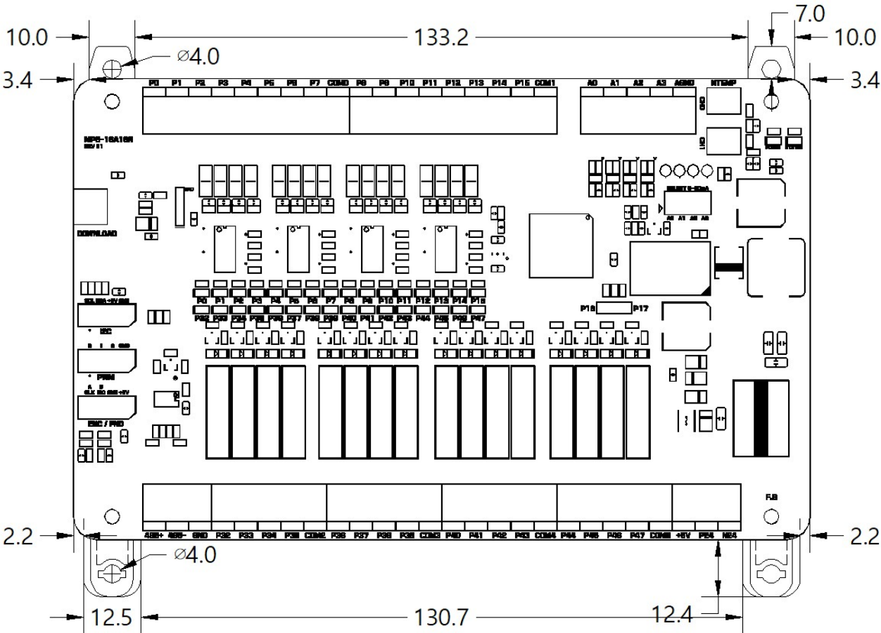
□ DIMENSION ( 클립 열었을 때 / 단레일 체결 전 )
