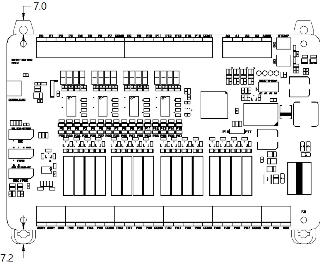
□ DIMENSION ( 클립 열었을 때 / 단레일 체결 후 )
