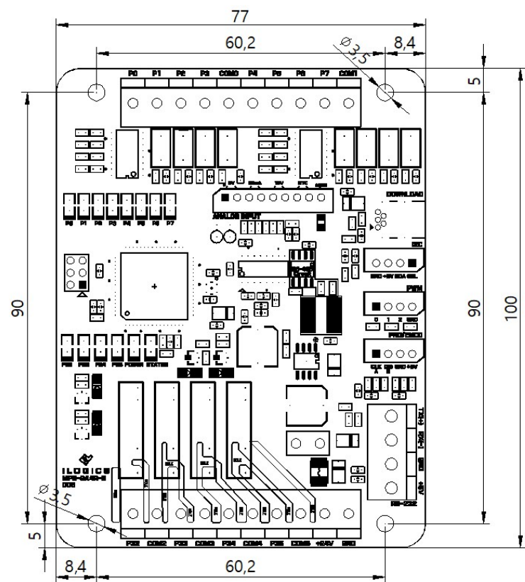
❑ DIMENSION ( PCB / 단레일 사용하지 않을 경우 )
