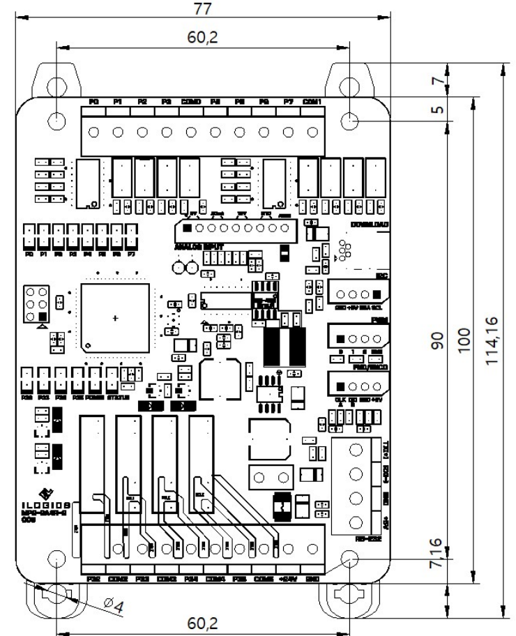
❑ DIMENSION ( 클립 닫았을 때 / 단 레일 체결 후 )
