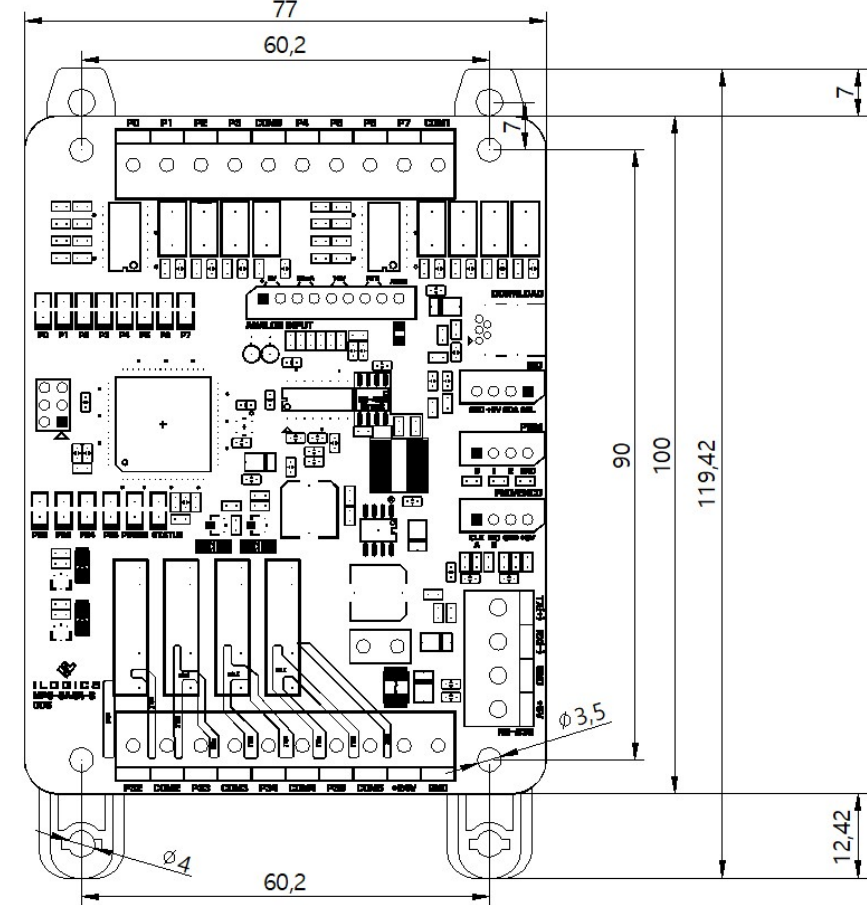
❑ DIMENSION ( 클립 열었을 때 / 단레일 체결 전 )
